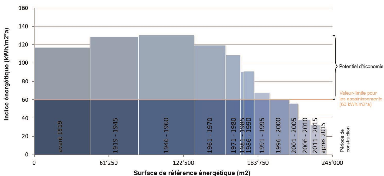
Figure 14 - Commune de Tavannes : Besoins de chaleur pour le chauffage des locaux d'habitation par période de construction, avec indice énergétique et surface de référence énergétique (SRE). Source: Données EBBE, 2020
