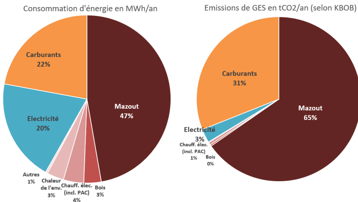
Figure 19 - Consommation d'énergie (20.1 MWh/hab.an) et émissions de GES (4.7 tCO 2 éq/hab.an) à Tavannes. Graphique: Jb.B
