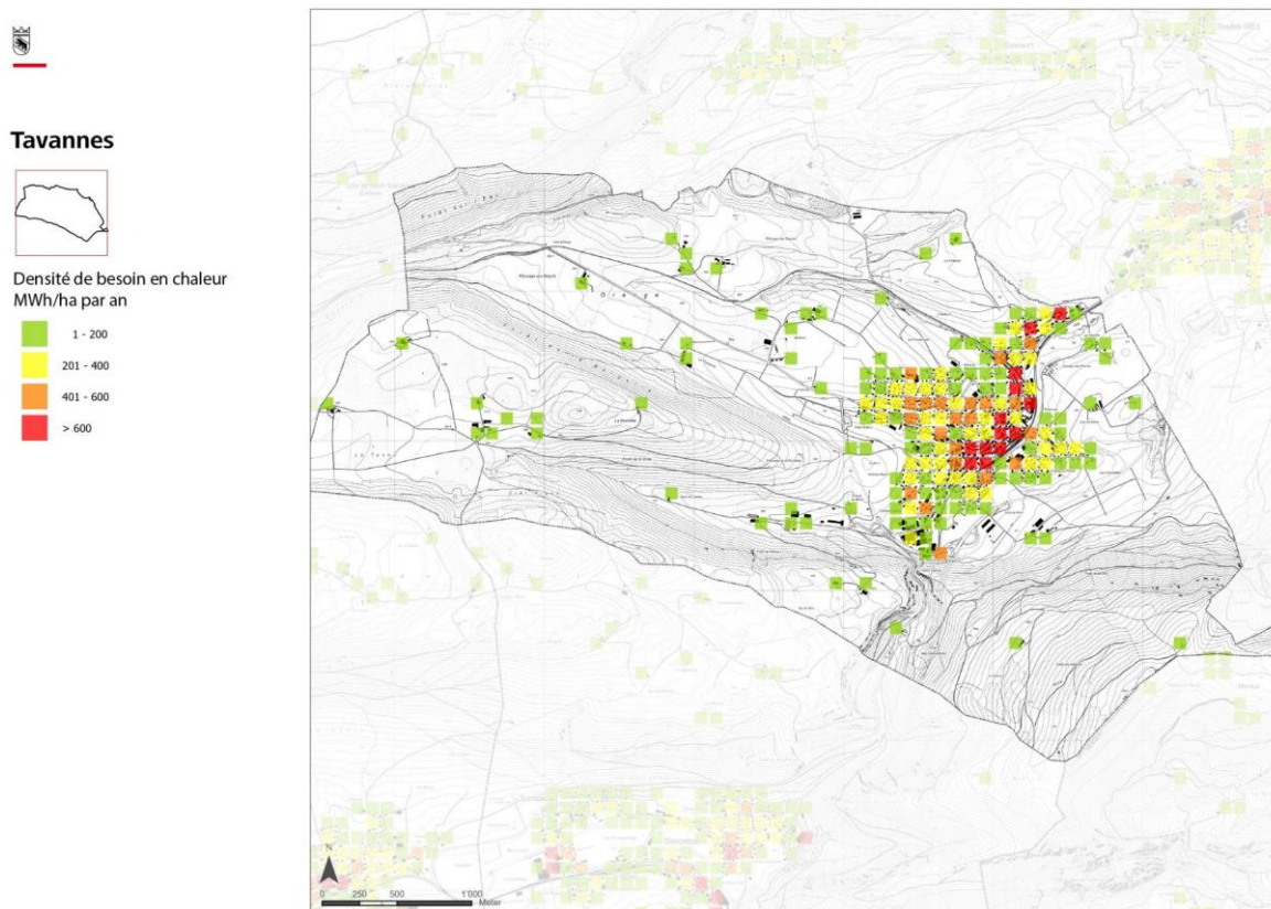
Figure 17 - Densité territoriale des besoins de chaleur de Tavannes. Chaque carré représente un hectare (surface de 100 x 100 m)
